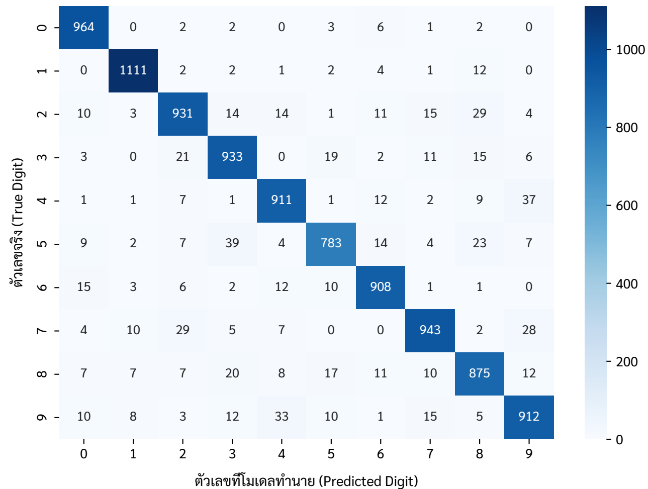
เมทริกซ์ความสับสน (Confusion Matrix, n=10,000)
