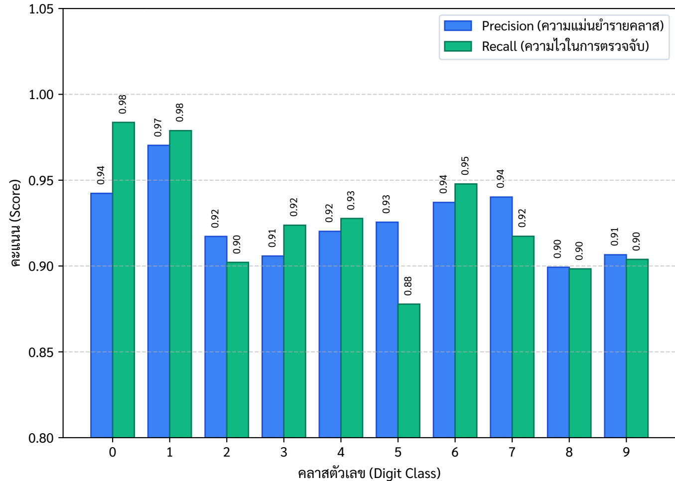
ค่า Precision และ Recall แยกตามคลาสตัวเลข 0-9
